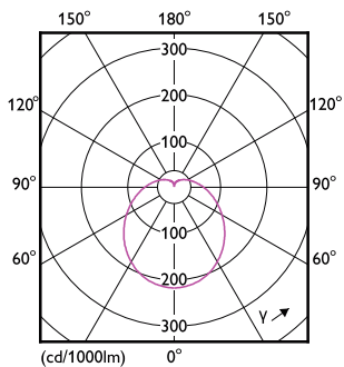
Light Distribution Diagram - 6A19/LED/830/FR/P/ND 1PF/6 NL
