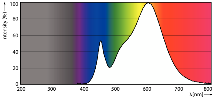
Spectral Power Distribution Colour - 6A19/LED/830/FR/P/ND 1PF/6 NL
