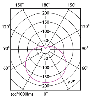
Light Distribution Diagram - 14A19/LED/865/FR/P/ND 1PF/6 NL
