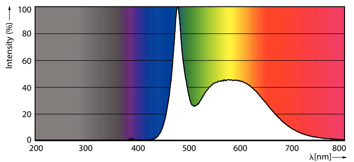
Spectral Power Distribution Colour - 14A19/LED/865/FR/P/ND 1PF/6 NL
