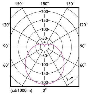
Light Distribution Diagram - 6A19/LED/865/FR/P/ND 1PF/6 NL
