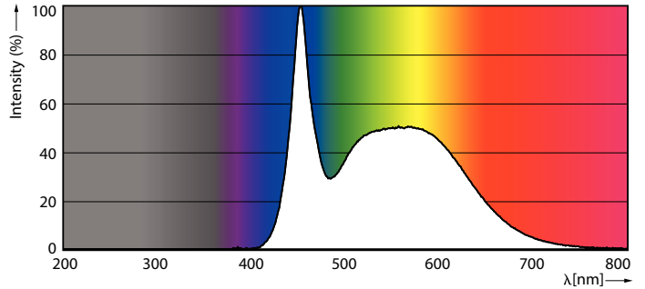
Spectral Power Distribution Colour - 6A19/LED/865/FR/P/ND 1PF/6 NL
